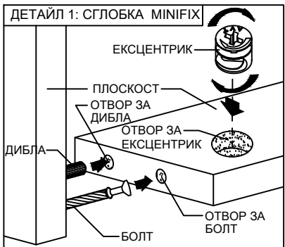
ДЕТАЙЛ 1: СГЛОБКА MINIFIX
