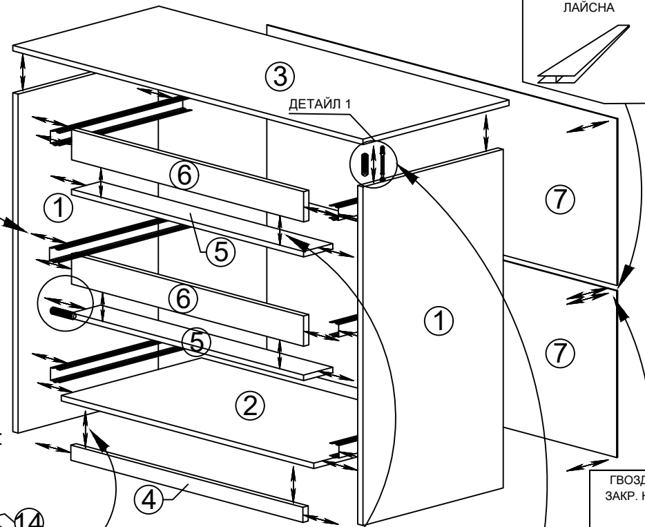
ДИБЛА - ЗА СГЛ. НА КОРПУСА
