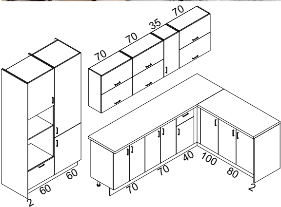
конфигурация №2 фронт: МДФ СУПЕР МАТ лате термоустойчив плот: дъб класик дължина на конфигурацията: 245см/187см/122см.
