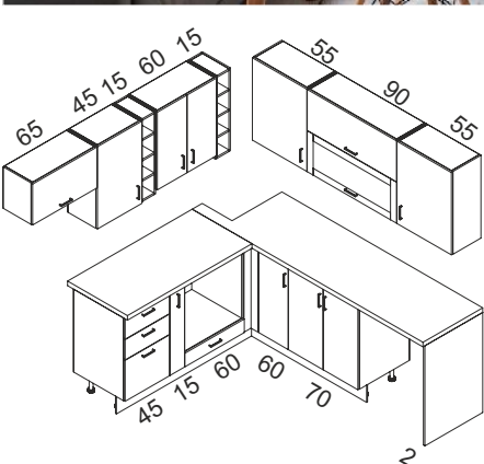
конфигурация №14 фронт: ПДЧ дъб крафт сив и ПДЧ бяло термоустойчив плот: бетон сив опал дължина на конфигурацията: 250см/230см.
