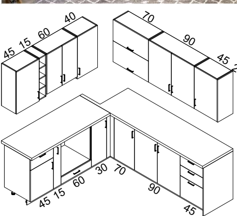
конфигурация №16 фронт: МДФ ГЛАНЦ зелен и МДФ ГЛАНЦ бял термоустойчив плот: тибур дължина на конфигурацията: 215см/257см.
