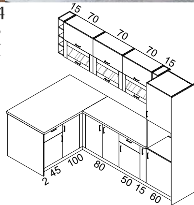
конфигурация №14 фронт: ПДЧ дъб крафт сив и ПДЧ бяло термоустойчив плот: бетон сив опал дължина на конфигурацията: 250см/230см.
